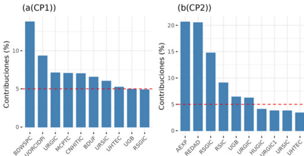
Figura 2. Contribución de las variables a los componentes principales a (CP1): contribución al componente principal 1, b (CP2): contribución al componente principal 2
