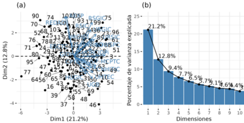
Figura 1. Componentes principales (a) y varianza explicada (b).
